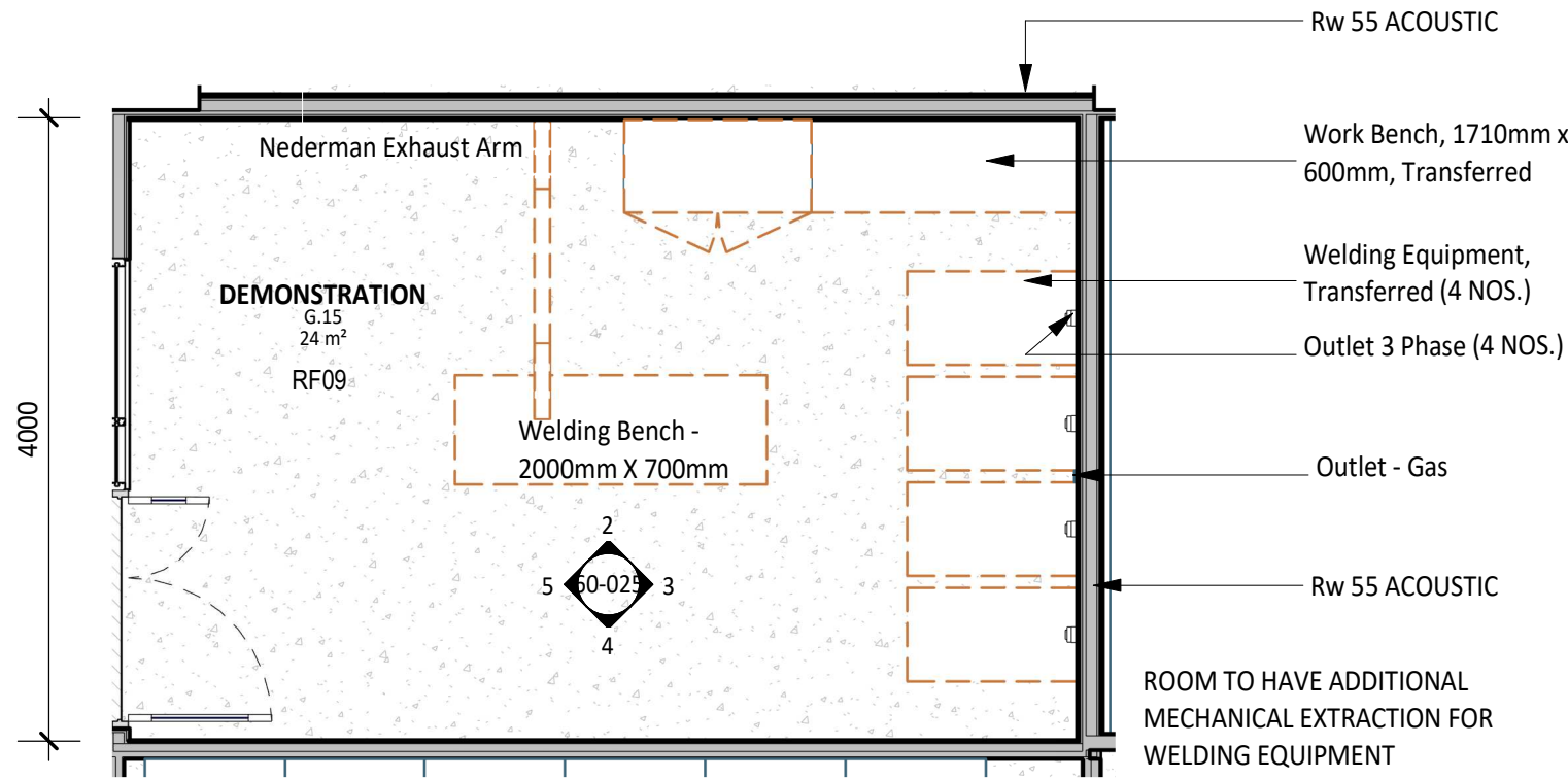
1 PLAN DETAIL 30-01 1 : 50
